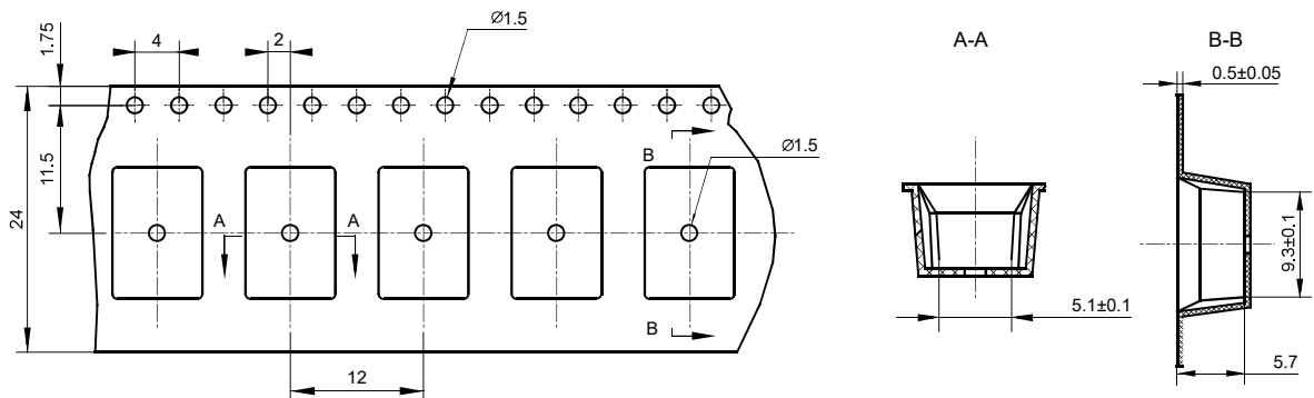
载带外形图
